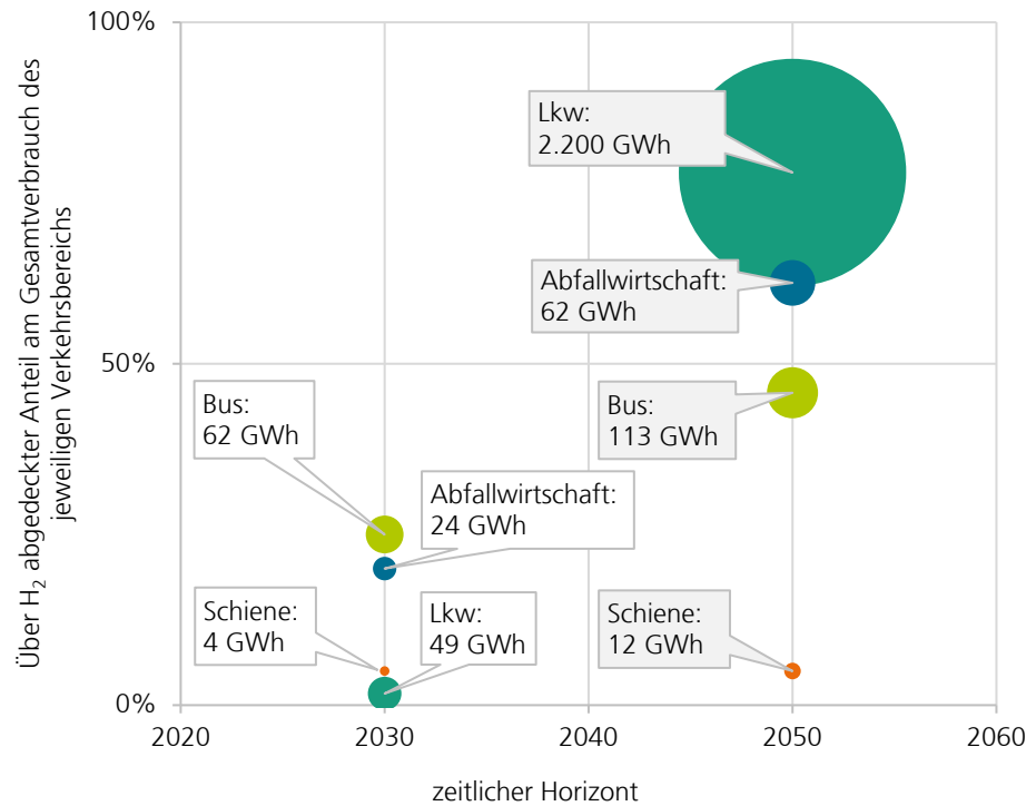
Abb. 07: Regionale Nachfrageentwicklung Wasserstoff im Verkehr.
